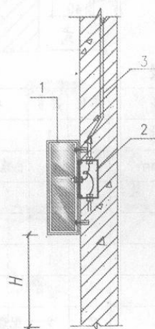
墙壁明装
