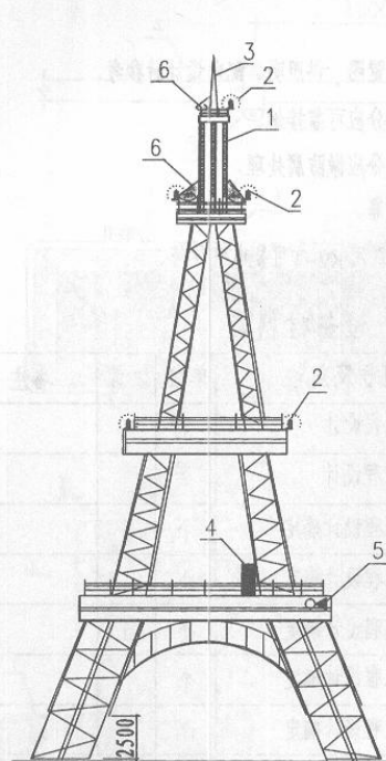
铁塔上线型光源灯具安装布置图
