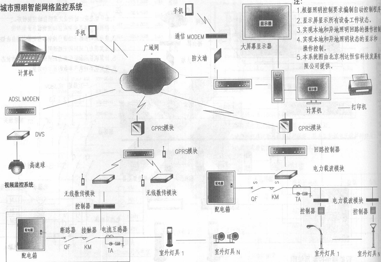
城市智能网络监控照明系统示意图
