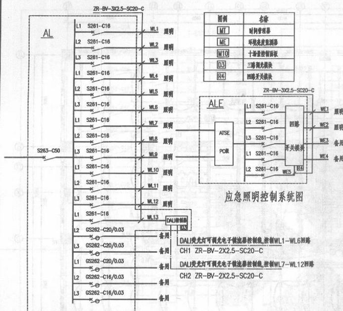
办公区照明控制系统图
