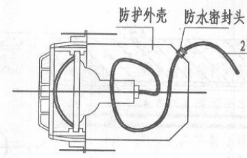
水下灯具结构一
