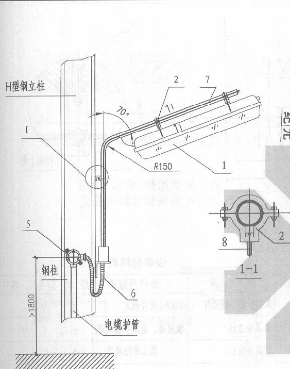
防护型荧光灯钢立柱上安装
