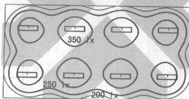
等照度曲线
