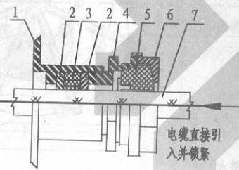
电缆布线引入装置
