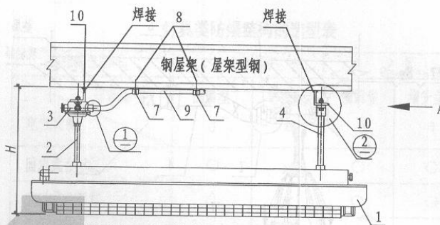
防爆(增安)吊杆荧光灯在钢屋架下安装
