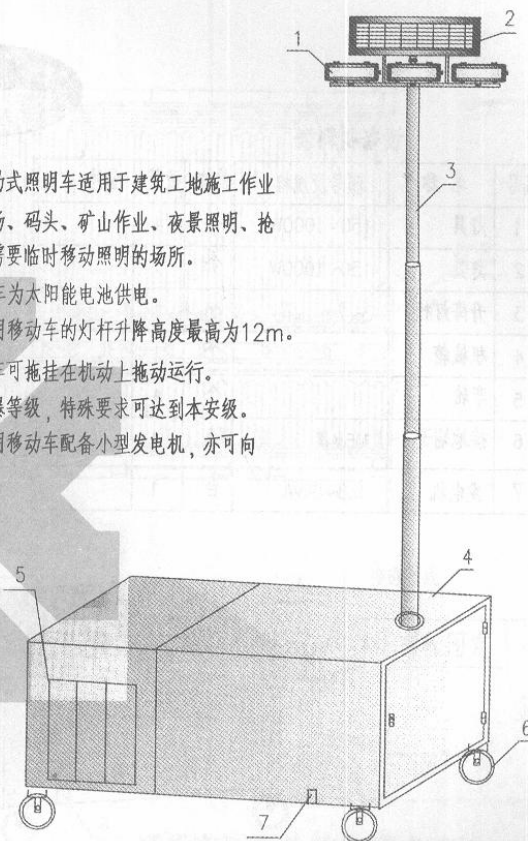
太阳能升降车灯示意图
