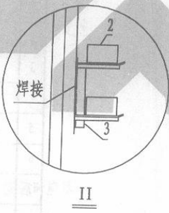
图名 投光灯在马道侧安装图
