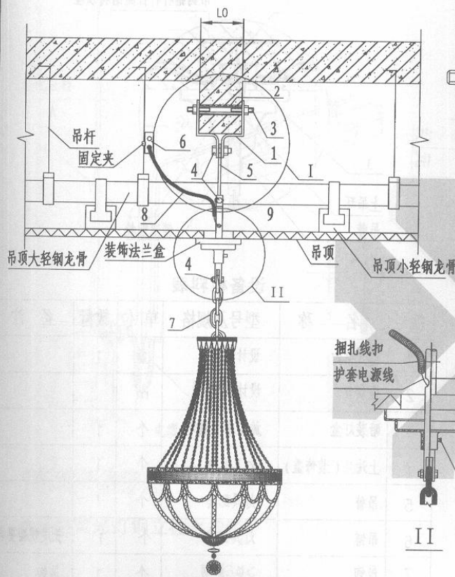
链式吊灯在吊顶下安装
