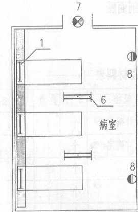
病室灯具布置平面
