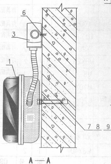
隧道灯安装示意图
