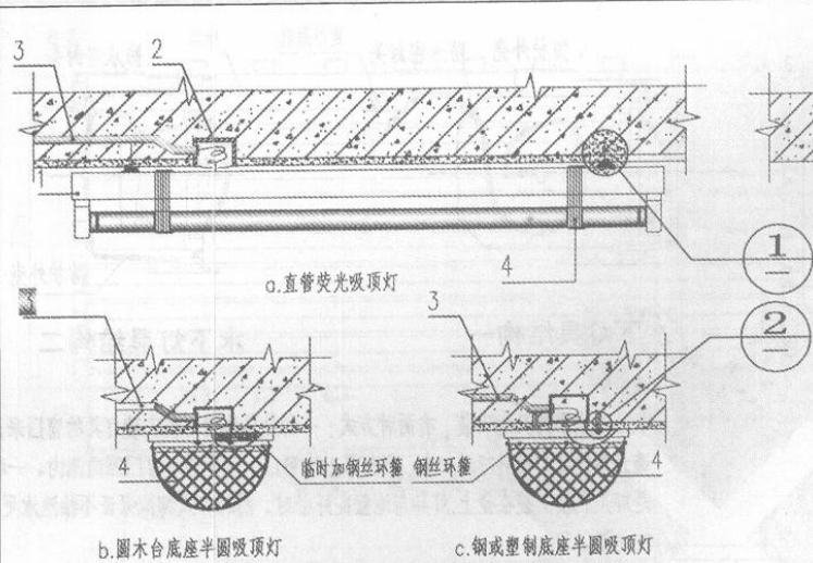
图一. 吸顶灯具安装示意图
