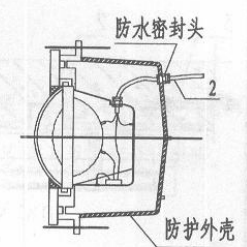
水下灯具结构二
