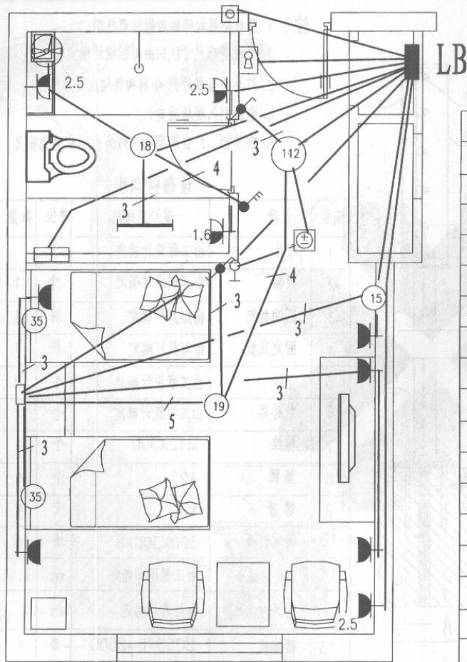
标准间放大平面
