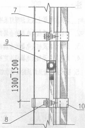
线型光源灯具抱箍式安装
