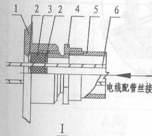
钢管布线引入装置
