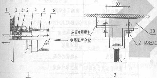
1. 防爆箱体 2. 金属垫圈 3. 密封圈 4. 压紧螺母 5. 电线护管 6. 电线
