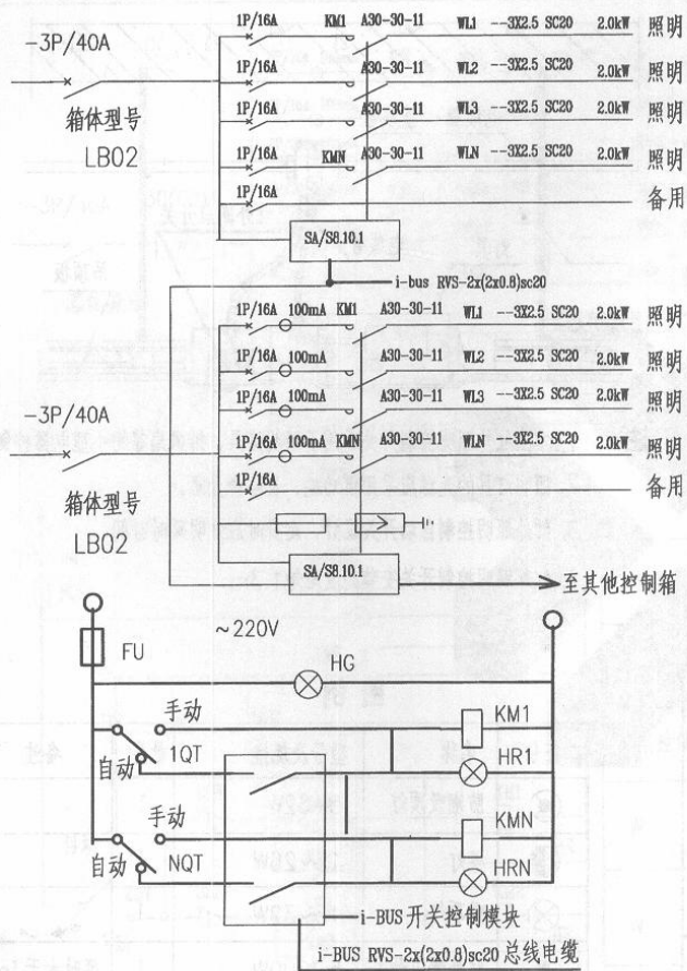
二次原理图
