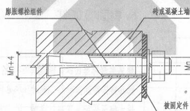
八式 墙上膨胀螺栓 Mn-螺栓直径
