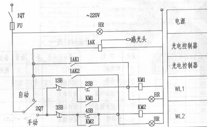
二次原理图
