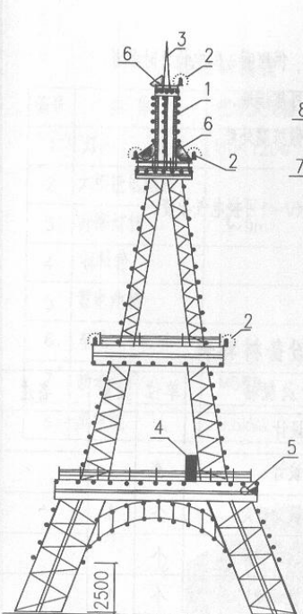
铁塔上点光源灯具安装布置图
