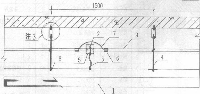
嵌入式荧光灯带安装图
