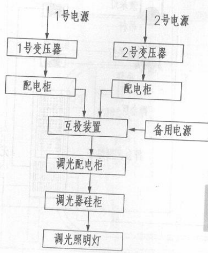
舞台调光系统供电方框图
