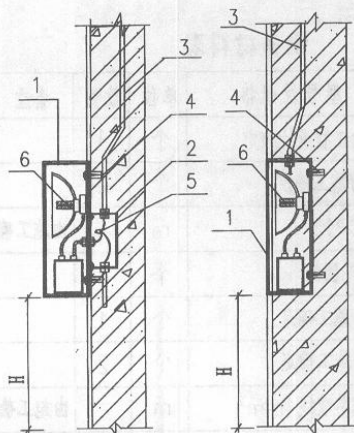
墙壁暗装 A—A
