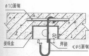
一式 现浇楼板预留吊环
