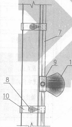
点光源灯具抱箍式安装
