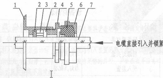
1. 隔爆壳体 2. 金属垫圈 3. 密封圈 4. 压紧螺母 5. 防脱封套 6. 防脱封盖 7. 电线
