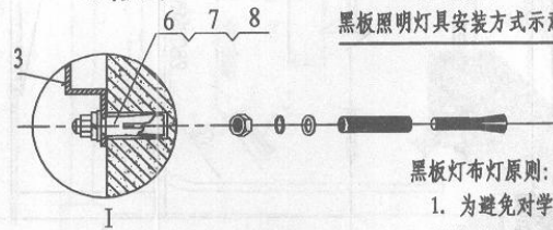
(a) 嵌入式
