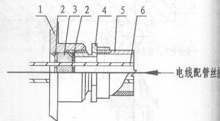
1. 隔爆壳体 2. 金属垫圈 3. 密封圈 4. 压紧螺母 5. 电线护管 6. 电线
