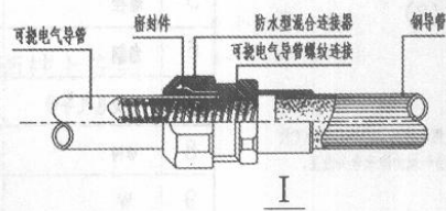
图 名 建筑立面泛光灯具安装图 图 集 号 09BD6 页 次 60
