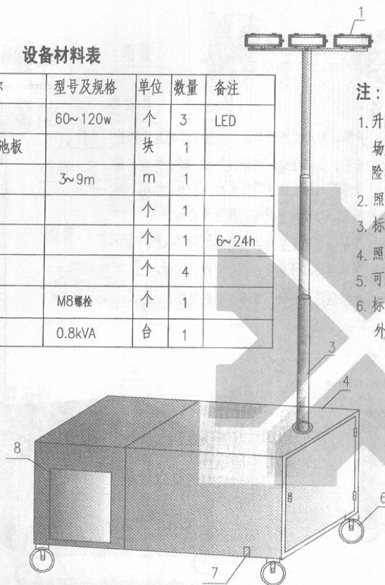
发电机升降车灯示意图
