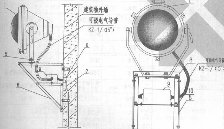
墙壁安装
