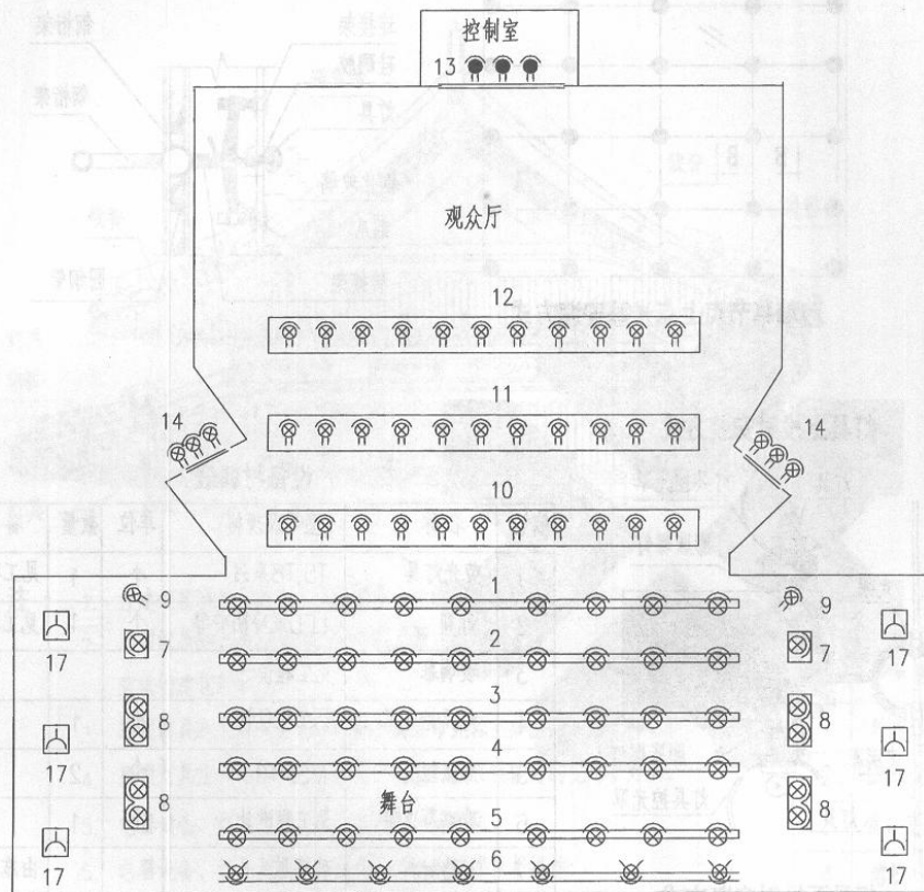
舞台灯具布置平面图
