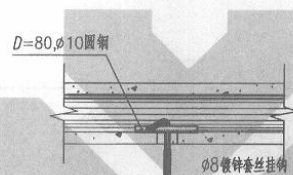
五式 圆孔预制楼板用挂钩螺栓
