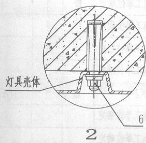
2. 双管盒式吸顶荧光灯在现浇混凝土屋面板下安装
