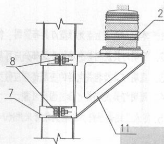
航空障碍灯抱箍式安装
