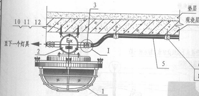
1. 吸顶安装 (钢管配线)
