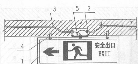
顶板安装
