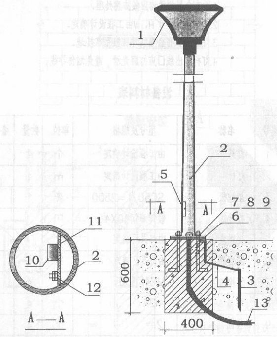
柱灯安装图
