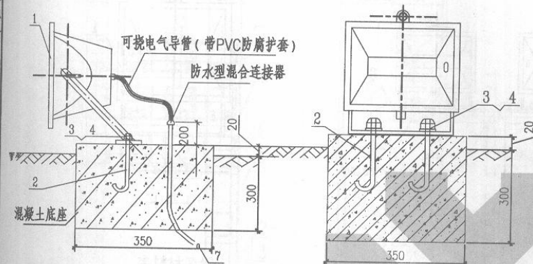
地面安装
