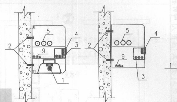
示例1 病床综合装置剖面图 示例2 病床综合装置剖面图
