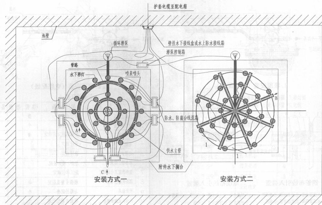
图 名 水中照明灯具安装图(一)
