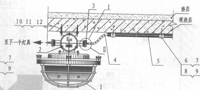
2. 吸顶安装 (电缆配线)
