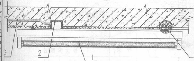
1. 单管盒式吸顶荧光灯在现浇混凝土屋面板下安装
